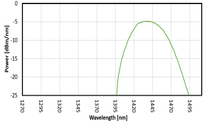
FIG. 2: SLED 1 SPECTRUM
