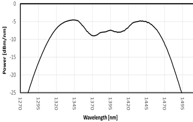
FIG. 1: ISB2 SPECTRUM
